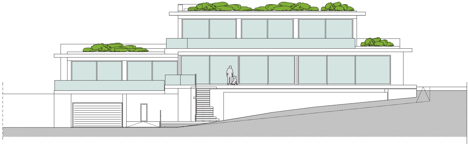
SOUTH SIDE | ALÇADO SUL
