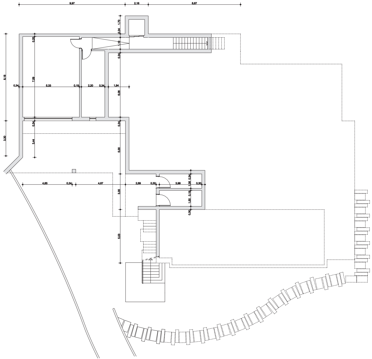
FLOOR -1 (GARAGE) | PISO -1 (GARAGEM)
